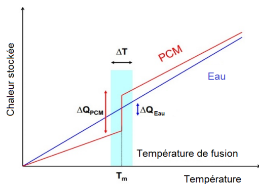
Figure 28: (À gauche) Alors que dans le cas du stockage de chaleur sensible (exemple de l'eau) la quantité de chaleur stockée est proportionnelle à la différence de température, la température reste constante lors du stockage de chaleur latente (MCP), qui implique un changement de phase (p. ex. solide/liquide). Dans ce cas, la chaleur est stockée dans l'énergie du changement de phase. (À droite) Exemple de stockage thermochimique (source de l'image: ZAE Bayern).
