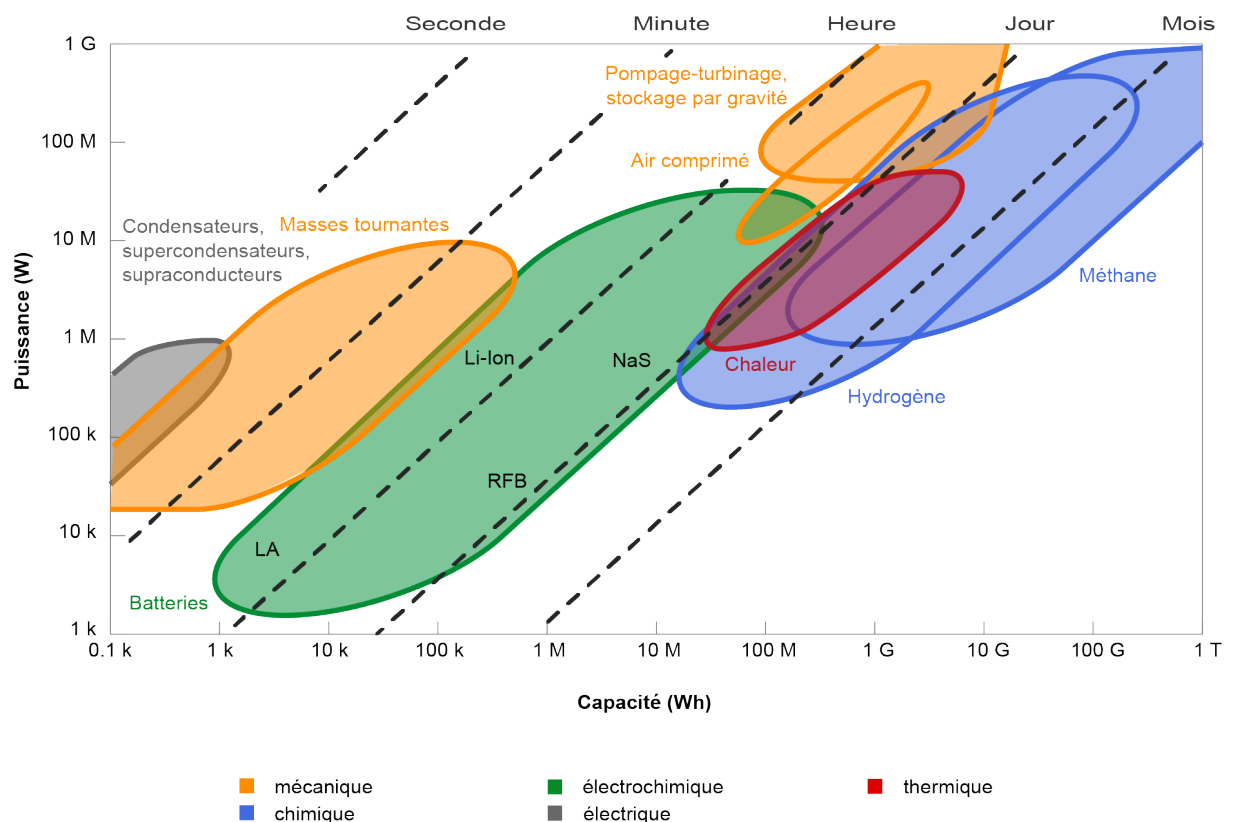
Figure 3: Aperçu schématique de la puissance et de l'énergie (capacité) des différents types de stockage (mécanique, chimique, électrochimique, électrique et thermique). Les temps de stockage possibles vont de quelques secondes à plusieurs mois. Les accumulateurs de chaleur et les réservoirs de gaz (hydrogène, méthane) sont intéressants en particulier pour le stockage d'énergie saisonnier sur plusieurs mois. (Li-Ion: batterie lithium-ion; NaS: batterie au sodium-soufre; LA: batterie au plomb ( lead-acid battery ); RFB: batterie à flux redox ( Redox-flow battery )).
