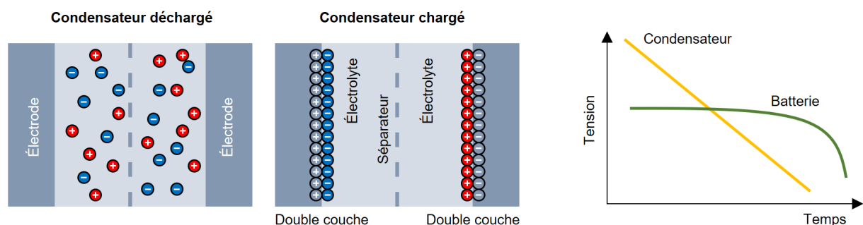
Figure 11: (À gauche) Principe d'un condensateur à double couche (supercondensateur). (À droite) Alors que les batteries peuvent fournir de l'énergie sur une longue période, on fait appel aux condensateurs en cas de besoin de puissances élevées sur de courtes périodes. Les supercondensateurs présentent une grande stabilité des cycles et une durée de vie relativement longue. Au cours des dernières années, d'importants progrès ont été réalisés sur le plan technologique et les supercondensateurs pourraient représenter une alternative au stockage par batterie en particulier dans le contexte industriel.
