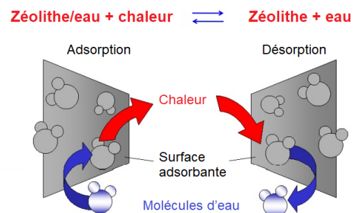
Figure 28: (À gauche) Alors que dans le cas du stockage de chaleur sensible (exemple de l'eau) la quantité de chaleur stockée est proportionnelle à la différence de température, la température reste constante lors du stockage de chaleur latente (MCP), qui implique un changement de phase (p. ex. solide/liquide). Dans ce cas, la chaleur est stockée dans l'énergie du changement de phase. (À droite) Exemple de stockage thermochimique (source de l'image: ZAE Bayern).
