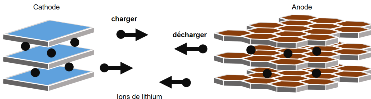
Figure 14: Dans les batteries lithium-ion, des ions de lithium sont échangés entre l'anode et la cathode pendant la charge et la décharge. La composition chimique des batteries se différencie en particulier par la structure de la cathode et de l'anode. La cathode est composée d'oxydes de métaux de transition (p. ex. lithium-nickel-manganèse-oxyde de cobalt) et l'anode de graphite (carbone).
