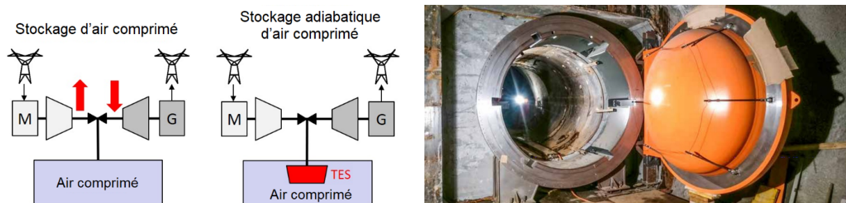
Figure 9: À gauche: le stockage d'air comprimé classique et adiabatique: l'électricité est prélevée du réseau, entraîne un compresseur au moyen d'un moteur (M) et l'énergie est stockée sous forme d'air comprimé dans le sous-sol. Dans le cas du stockage adiabatique d'air comprimé, la chaleur dégagée est stockée dans un accumulateur thermique (AT). Lors de l'évacuation, l'air comprimé se détend à travers une turbine et produit de l'électricité grâce à un générateur (G). (À droite) Galeries de test au Gothard (source de l'image: ALACAES, https://alacaes.com ).
