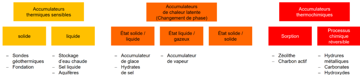
Figure 26: Classification des différents types de stockage thermique: (1) accumulateurs thermique sensibles, (2) accumulateurs de chaleur latente, (3) accumulateurs thermochimiques (avec quelques exemples).
