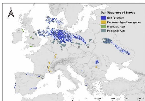
Figure 23: (À gauche) Gisements de sel et structures salines européens ressortant de l'évaluation de l'aptitude au stockage souterrain d'hydrogène. (À droite) Potentiel global de stockage en cavité dans les pays européens en fonction des critères «onshore», «offshore» et «onshore à moins de 50 km des côtes» ( https://doi.org/10.1016/j.ijhydene.2019.12.161 ).
