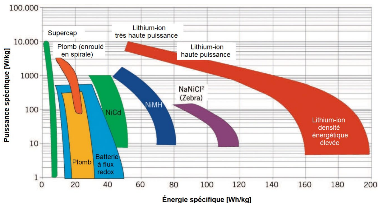
Figure 13b: Diagramme de Ragone: technologies de batterie selon leur densité de puissance (W/kg) et leur densité énergétique (Wh/kg).
