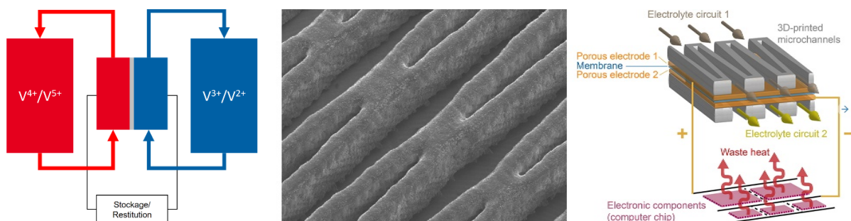
Figure 20: (À gauche) Principes d'une batterie à flux redox. (À droite) Dans le cadre d'un projet de recherche sur trois ans, le laboratoire de recherche d'IBM à Zurich a développé une technologie de flux redox destinée au refroidissement et à l'alimentation de puces électroniques. L'image du milieu montre les micro-canaux par lesquels l'électrolyte est amené vers la puce.
