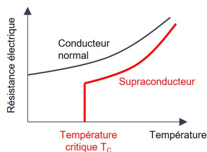
Figure 12: (À gauche) Au-dessous d'une certaine température (température de transition), les supraconducteurs ne présentent aucune résistance électrique. Il est possible de construire des accumulateurs électriques à l'aide de bobines supraconductrices en stockant l'énergie dans le champ magnétique des bobines. (À droite) Découverts dans les années 80 (prix Nobel de physique en 1987 pour les chercheurs Müller et Bednorz du centre de recherche d'IBM, https://link.springer.com/content/pdf/10.1007/BF01303701.pdf ), les supraconducteurs à haute température affichent des températures critiques de l'ordre de 90 K et plus. Photo: un aimant volant au-dessus d'un supraconducteur à haute température pour illustrer l'état supraconducteur (effet Meissner-Ochsenfeld).
