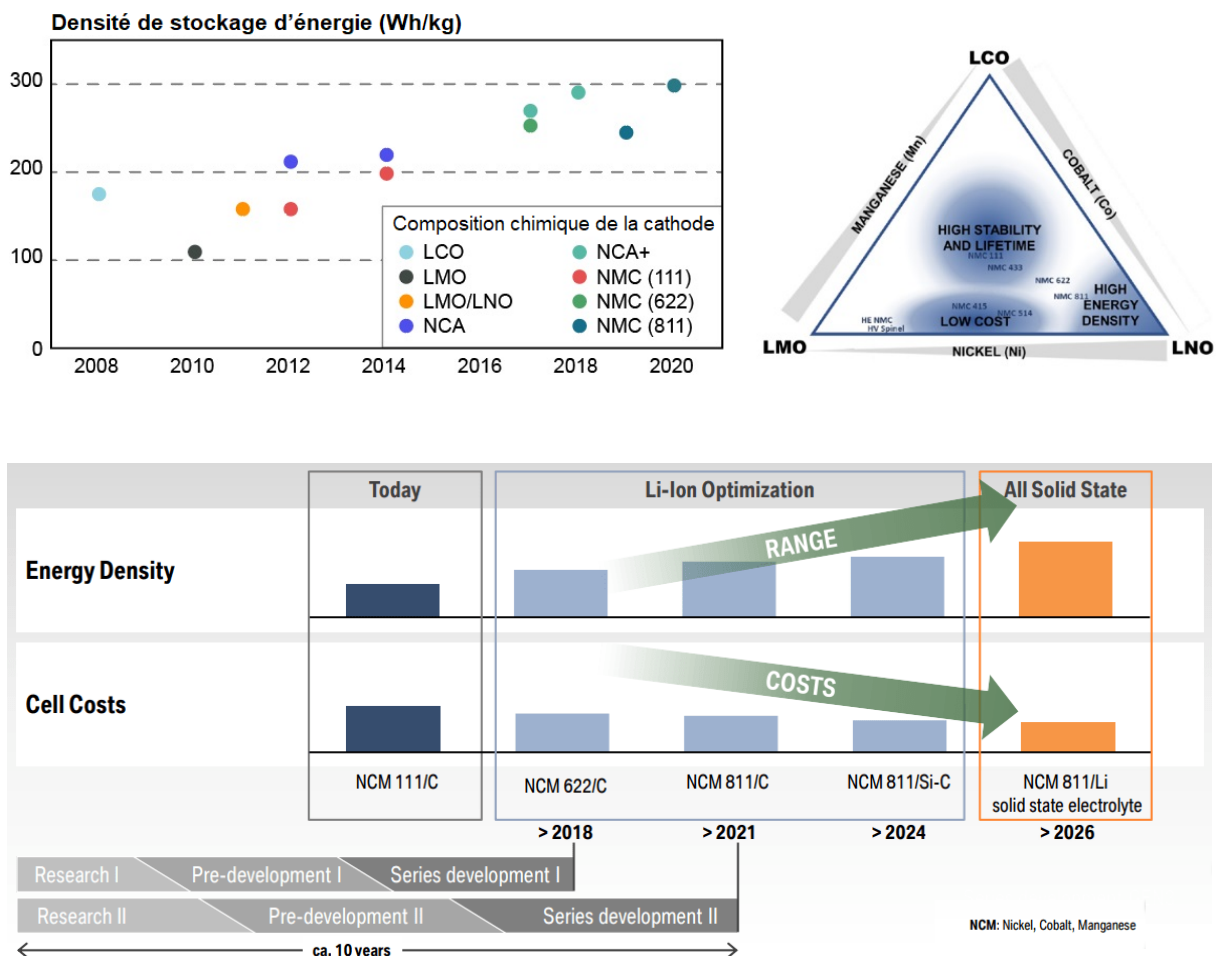
Figure 15: (En haut à gauche) Au cours des dernières années, la densité de stockage des batteries lithium-ion a presque triplé (source: BloombergNEF, 2020). (En haut à droite) En ce qui concerne la technologie NMC, la stabilité, la durée de vie, les coûts, la densité énergétique et la durabilité dépendent de la composition des différents éléments (nickel, manganèse et cobalt). Depuis quelques années, le nickel remplace de plus en plus le cobalt. (En bas) Feuille de route simplifiée de la technologie de batterie lithium-ion (source: BMW Group, 2016).
