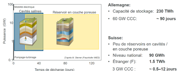
Figure 22: (À gauche) Le stockage d'hydrogène et de méthane synthétique à grande échelle sur de longues périodes nécessite des espaces de stockage souterrains. Les cavités salines et les réservoirs en couche poreuse se prêtent à cette utilisation. Alors que ce type de grand réservoir est disponible ou pourrait être construit ailleurs en Europe, il n'existe pas encore vraiment de telles possibilités de stockage en Suisse. (À droite) Il est relativement facile de construire des cavernes artificielles dans des roches salines. Sur la photo: une mine de sel en Roumanie. Une étude récente de la RWTH Aachen ( https://doi.org/10.1016/j.ijhydene.2019.12.161 ) évalue la capacité de stockage totale de l'hydrogène en Europe à 84,8 petawattheures (PWh). À titre de comparaison, le potentiel total du pompage-turbinage en Europe est d'environ 0,12 PWh et la consommation d'énergie primaire en Suisse s'élève à 0,3 PWh.
