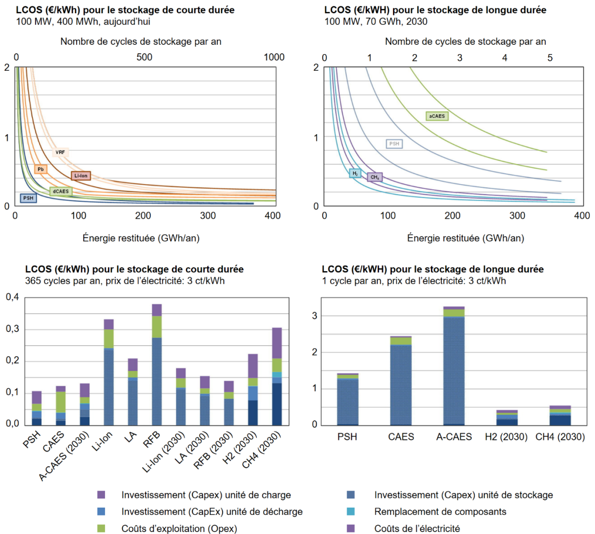
Figure 2b: (En haut) Levelized Cost of Storage LCOS (coût de stockage nivelé) pour le stockage de courte ou de longue durée par rapport à l'énergie restituée et au nombre de cycles par an. (En bas) LCOS pour le stockage de courte ou de longue durée pour différentes technologies: PSH: pompage-turbinage; CAES: stockage d'air comprimé ( Compressed Air Energy Storage ); A-CAES: stockage adiabatique d'air comprimé ( Adiabatic Compressed Air Energy Storage ); Li-Ion: batteries lithium-ion; LA: batteries au plomb; RFB: batterie à flux ( Redox-flow battery ); H2: stockage souterrain d'hydrogène; CH4: méthane synthétique (stockage souterrain). Pour la description des différentes technologies, voir le chapitre suivant.
