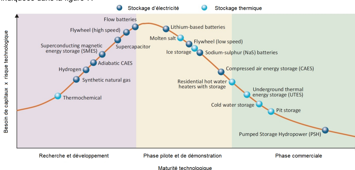
Figure 7: Différentes technologies de stockage d'électricité et de chaleur à divers degrés de développement (source: AIE, Technology Roadmap Energy Storage).
