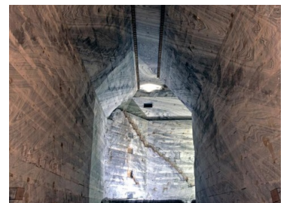
Figure 22: (À gauche) Le stockage d'hydrogène et de méthane synthétique à grande échelle sur de longues périodes nécessite des espaces de stockage souterrains. Les cavités salines et les réservoirs en couche poreuse se prêtent à cette utilisation. Alors que ce type de grand réservoir est disponible ou pourrait être construit ailleurs en Europe, il n'existe pas encore vraiment de telles possibilités de stockage en Suisse. (À droite) Il est relativement facile de construire des cavernes artificielles dans des roches salines. Sur la photo: une mine de sel en Roumanie. Une étude récente de la RWTH Aachen ( https://doi.org/10.1016/j.ijhydene.2019.12.161 ) évalue la capacité de stockage totale de l'hydrogène en Europe à 84,8 petawattheures (PWh). À titre de comparaison, le potentiel total du pompage-turbinage en Europe est d'environ 0,12 PWh et la consommation d'énergie primaire en Suisse s'élève à 0,3 PWh.
