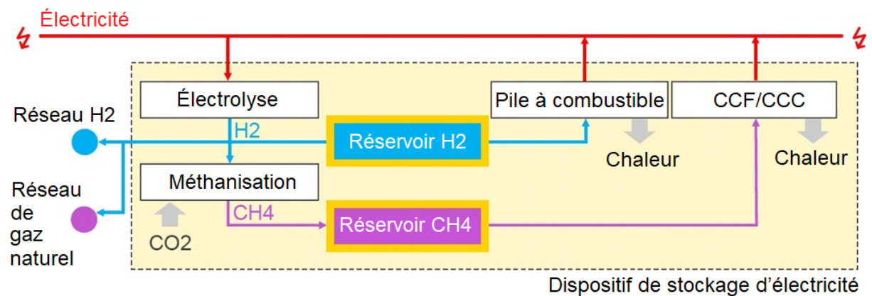
Figure 21: Le concept du Power-to-Gas en tant que système de stockage (CCF = couplage chaleur-force, CCC = centrales à gaz à cycle combiné).
