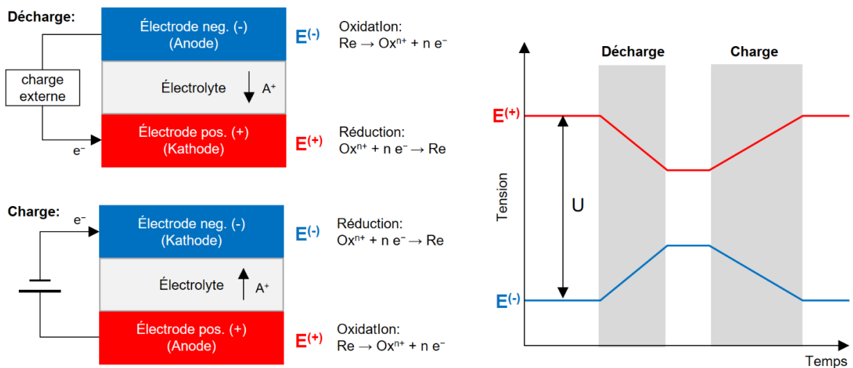
Figure 13a : Réactions électrochimiques lors de la décharge et de la charge de batteries (accumulateurs). La tension U d'une batterie résulte de la différence de potentiel électrochimique E des deux électrodes (demi-cellules), qui sont reliées entre elles par un électrolyte conducteur d'ions ( A^+ ). Pendant le processus de décharge, l'anode est oxydée et libère des électrons ( e^- ) ( n = nombre d'électrons), qui atteignent la cathode via une charge externe (par exemple, un moteur électrique) pour y réduire la cathode ( Re = état réduit, Ox = état oxydé).
