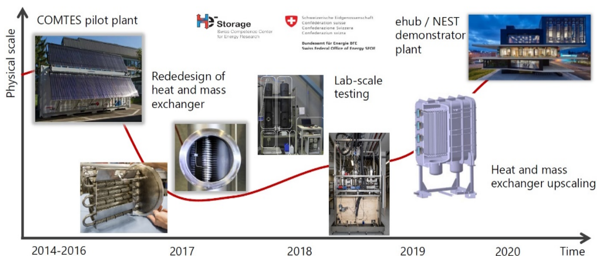
Figure 29: Au cours des dernières années, des progrès technologiques ont été réalisés en Suisse dans le domaine du stockage de chaleur thermochimique saisonnier utilisant des matériaux d'absorption liquides dans le cadre de projets européens et de l'OFEN et en collaboration avec le centre compétence SCCER «Heat and Electricity Storage» (L. Baldini, Empa und P. Gantenbein, OST, 2021).
