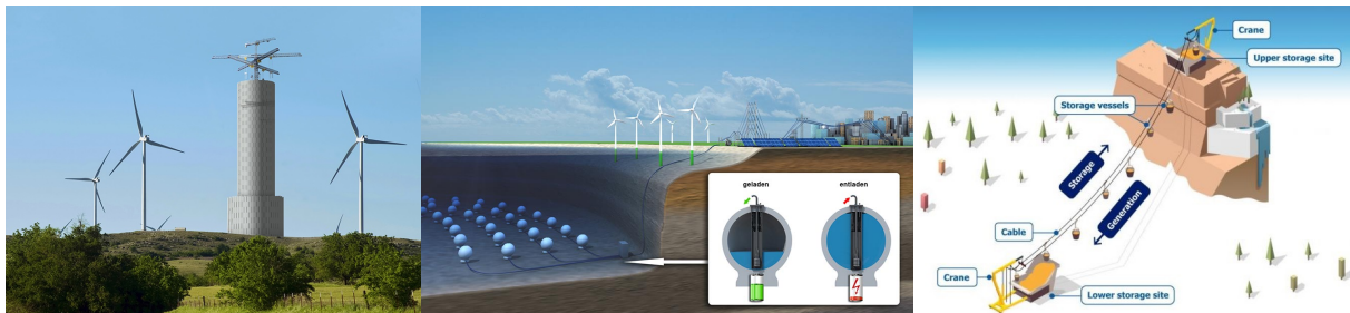
Figure 8: (À gauche) Technologie de stockage d'énergie de l'entreprise Energy Vault, qui empile des blocs de 35 tonnes composés de débris de construction compressés (source: Energy Vault). (Milieu) Le principe du stockage d'énergie par gravité qui utilise des sphères creuses immergées est semblable à celui d'une centrale de pompage-turbinage classique (source de l'image: Fraunhofer IWES, www.iwes.fraunhofer.de ). (À droite) Concept du Mountain Gravity Energy Storage de l'International Institute for Applied Systems Analysis (IIASA) (source de l'image: IIASA).
