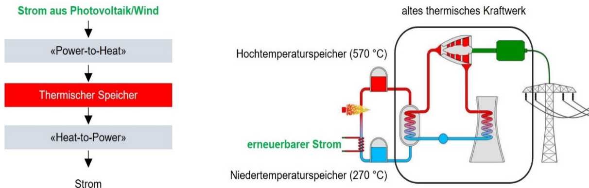
Figure 30: Principe très schématique de la batterie Carnot: l'électricité est utilisée pour produire de la chaleur à haute température directement par résistance ou lors d'un cycle thermodynamique. En cas de demande, un cycle thermodynamique permet également de produire de l'électricité en utilisant éventuellement une infrastructure existante (ancienne centrale thermique). (À droite: schéma du Centre allemand pour l'aéronautique et l'astronautique DLR).
