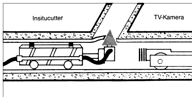
Abb. 3.17 Auffräsen des seitlichen Anschlusses mittels Cutter.
