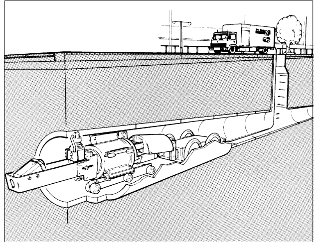
Abb. 4.4 Instandsetzung durch Reparatur mittels Kanal-Roboter.
