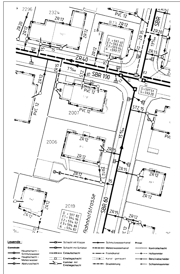
Abb. 2.1 Korrekt nachgeführte Kanalisationskataster gehören zu den wichtigsten Projektgrundlagen.
