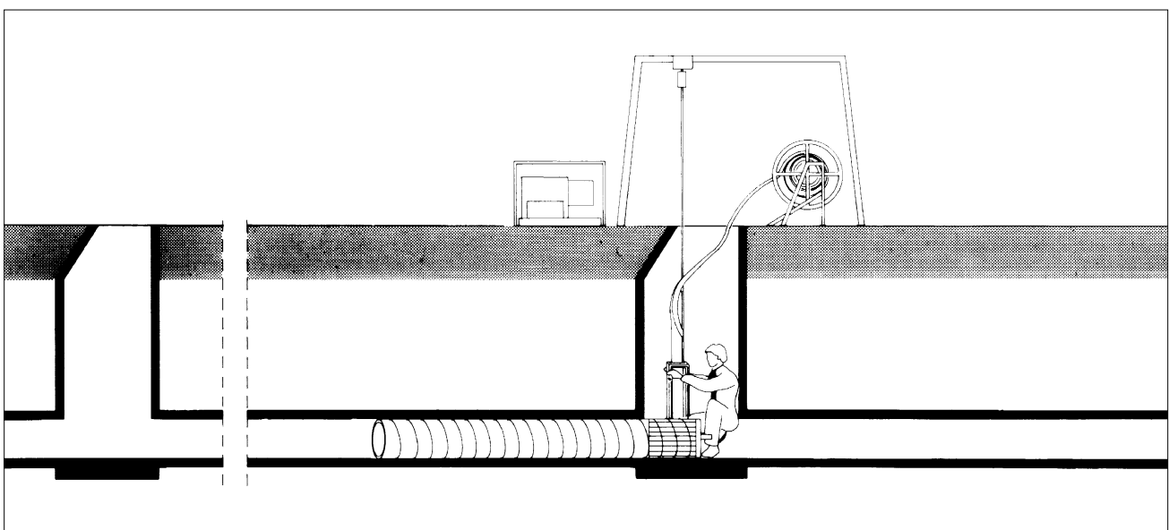
Abb. 4.13 Wickeln und Verschieben des Spiralrohres beim Wickelrohr-Relining.
