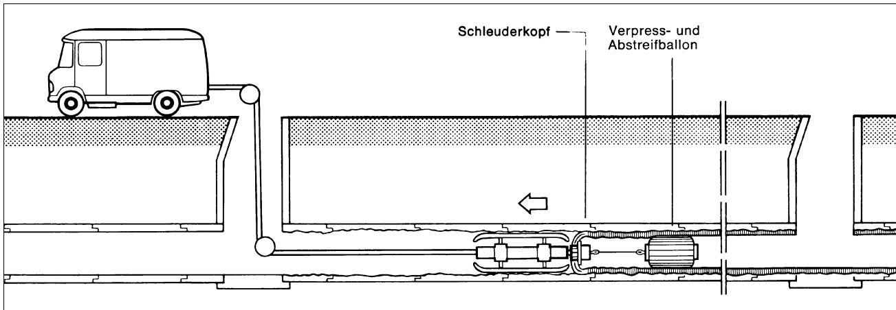
Abb. 4.9 Beschichtung mit Zementmörtel.
