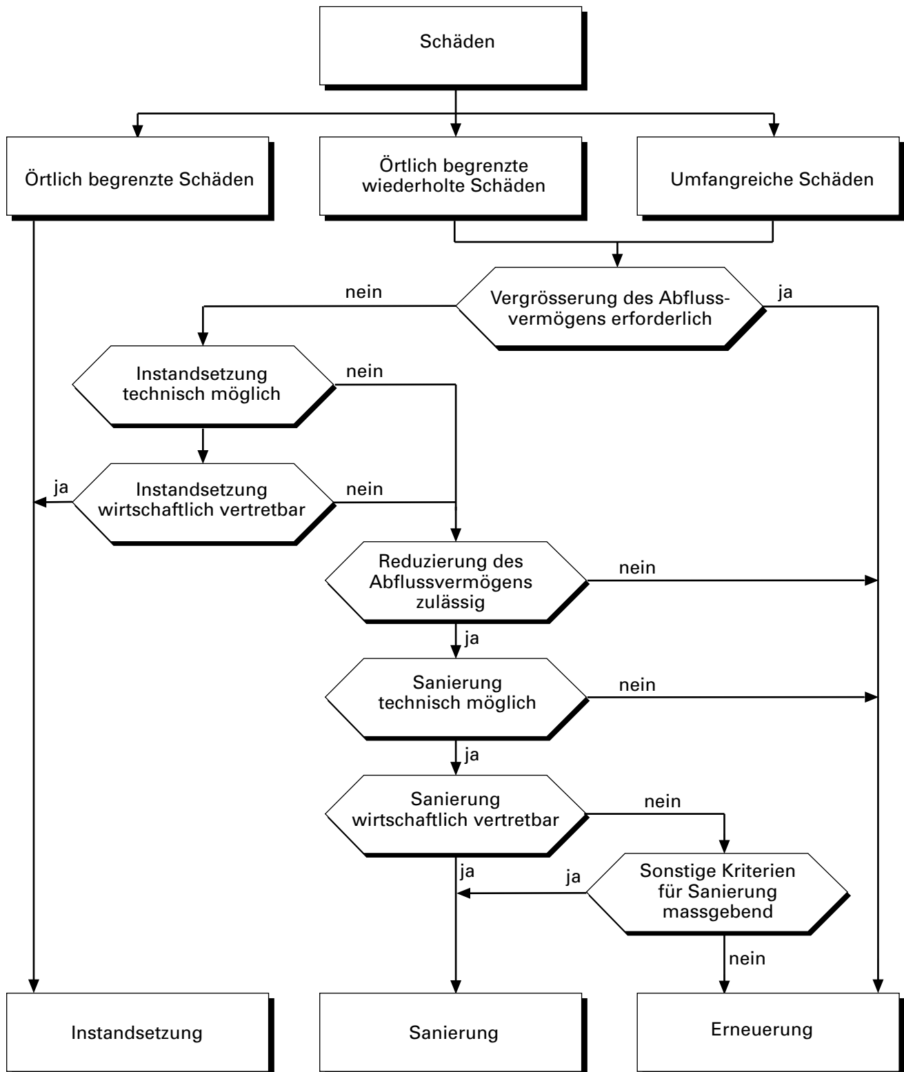
Abb. 5.1 Ablauf des Entscheidungsprozesses zur Wahl der geeigneten Verfahrensgruppe (Instandsetzung, Sanierung, Erneuerung).
