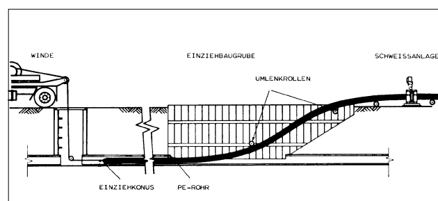
Abb. 4.10 Einziehen des Rohres beim Rohrstrang-Relining.
