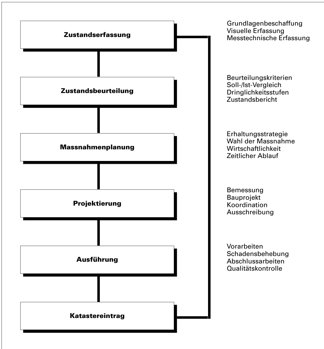
Abb. 3.2 Arbeitsablauf bei der Kanalisationserhaltung mit Vorgehensschritten und Einzelleistungen.
