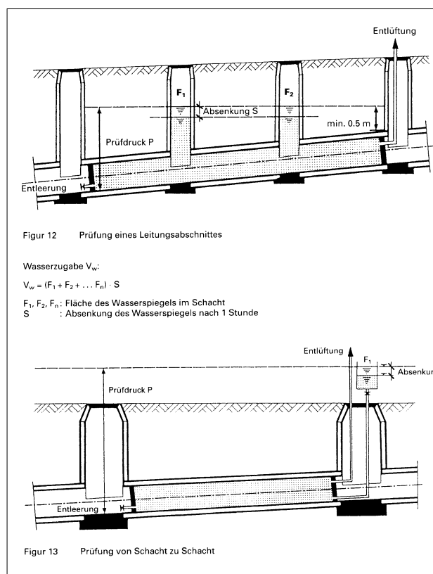
Abb. 3.19 Dichtigkeitsprüfung mit Wasser nach der SIA-Empfehlung V 190.
